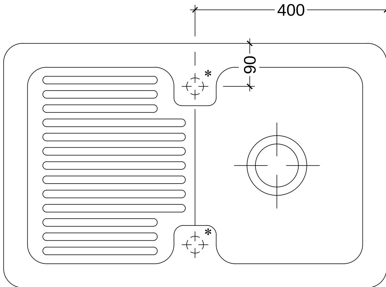
Spüle - CONDOR 45 Art. 6745 01 / 02
